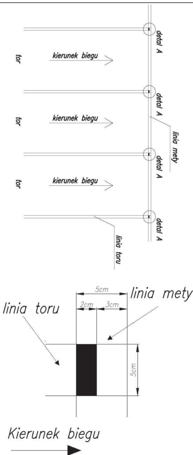
Rys. Schemat wyznaczania na linii mety oznaczeń do kontroli prawidłowości ustawienia
