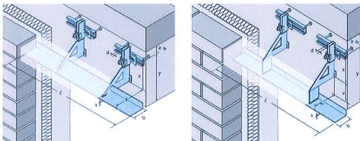
Rys. Przykładowe zastosowanie wsporników pod elewacje ceglane.
