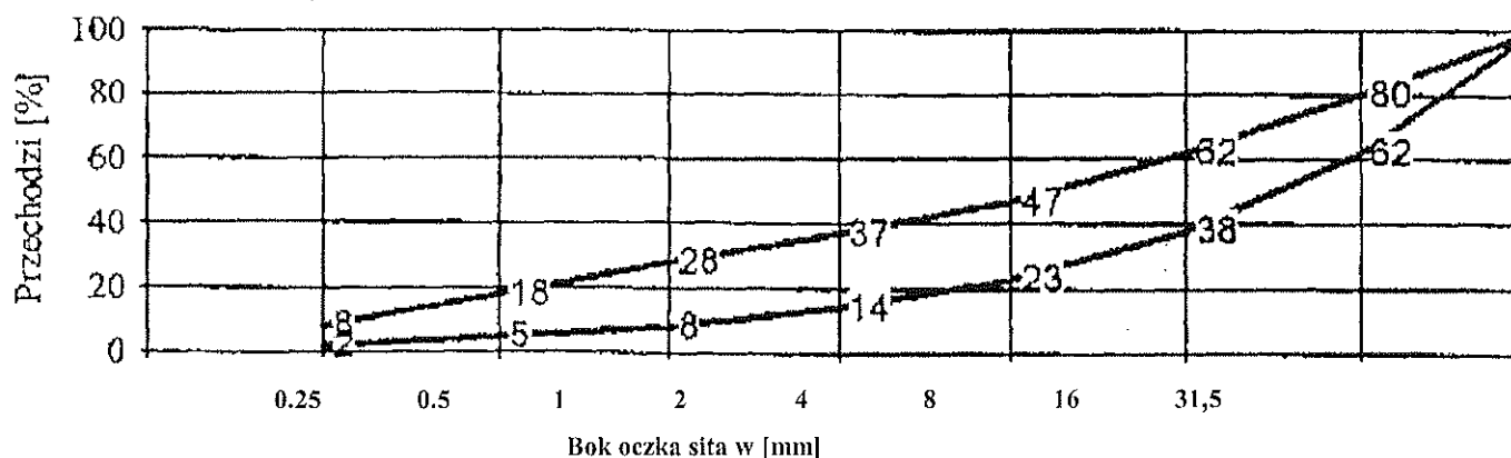
Krzywa uziarnienia kruszyw 0-31,5 mm
