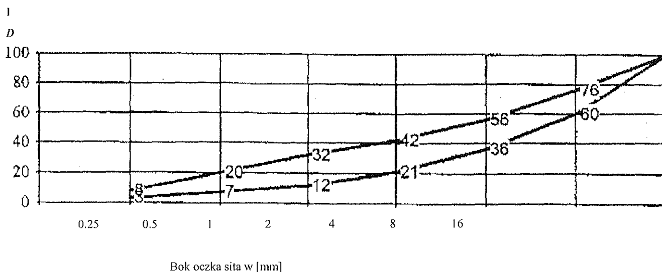
Krzywa uziarnienia kruszyw 0 - 16 mm
